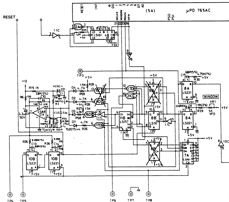
Fig. 2-22 VFO Circuit
